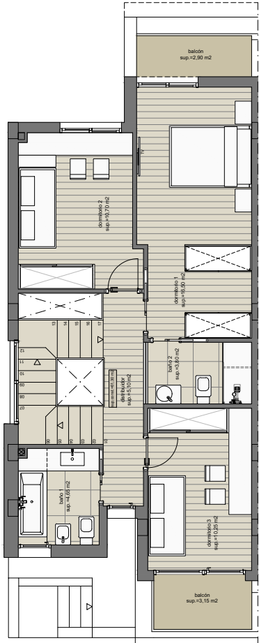
Planta PRIMERA, Vivienda Tipo B4.
