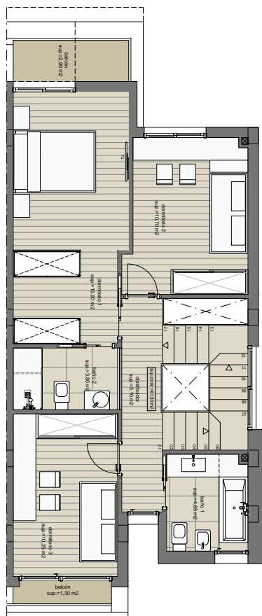
Planta PRIMERA. Vivienda Tipo B4.2.
