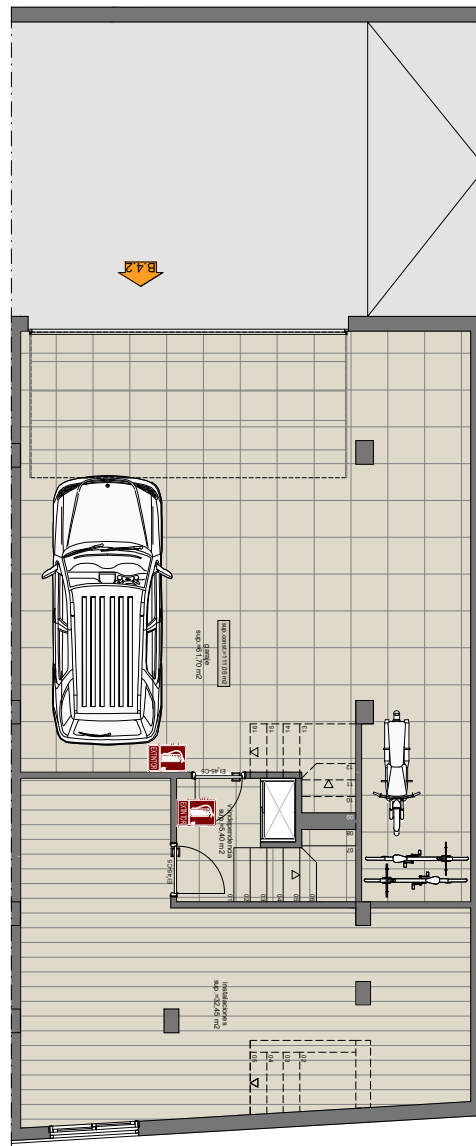
Planta BAJA. Vivienda Tipo B4.2.
